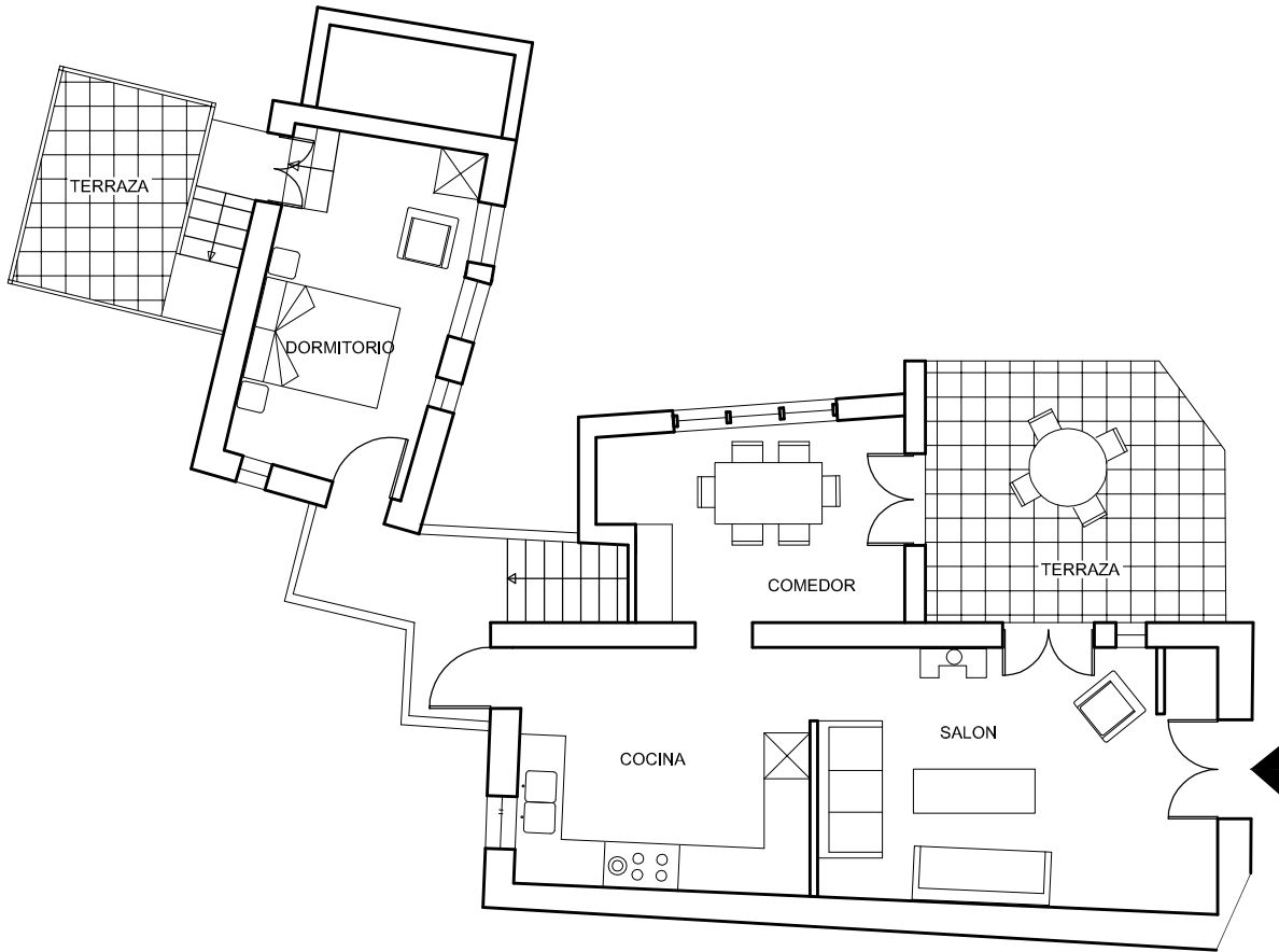
PLANTA ALTA
